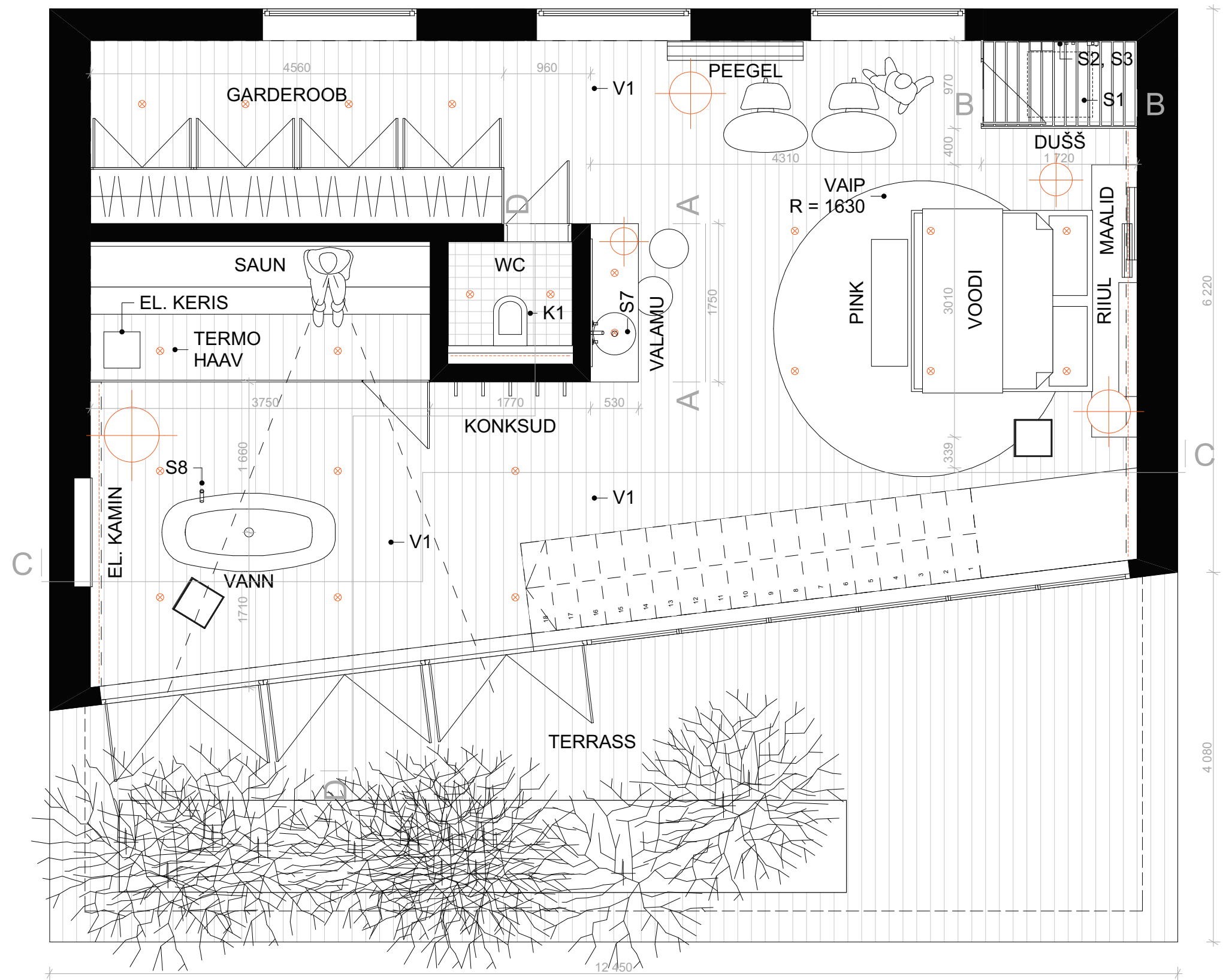
PLAAN M 1:50
